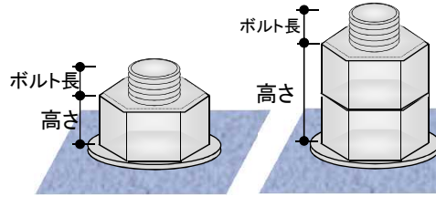
ナットキャップ NCPW スッポリキャップ SCPW 2ピースネジカバー 2PNCW
